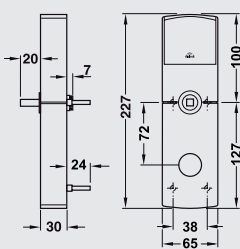
Зовнішній модуль
